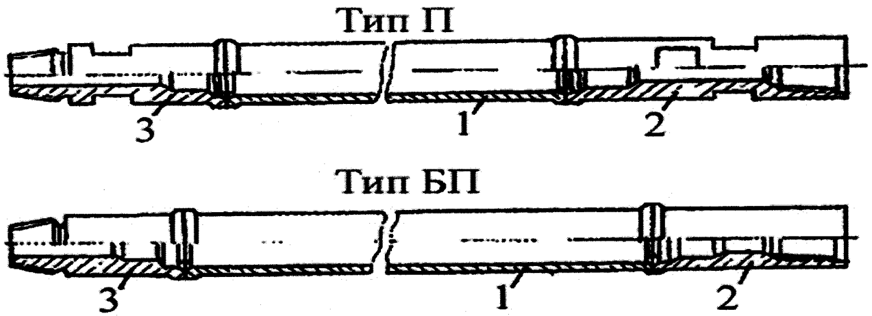
Рис. 133.3 Внешний вид бурильных труб
