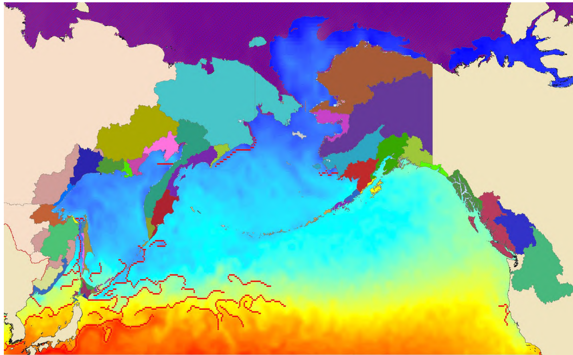
Фронтальные зоны (градиент 1^{\circ}\text{C} и более) на 03 ноября 2025 года
